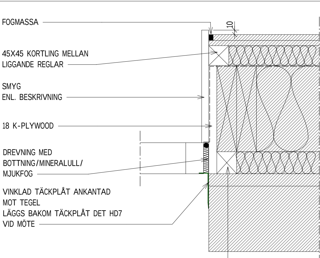
HD6 PRINCIPDETALJ 1:5 METALLPARTI
