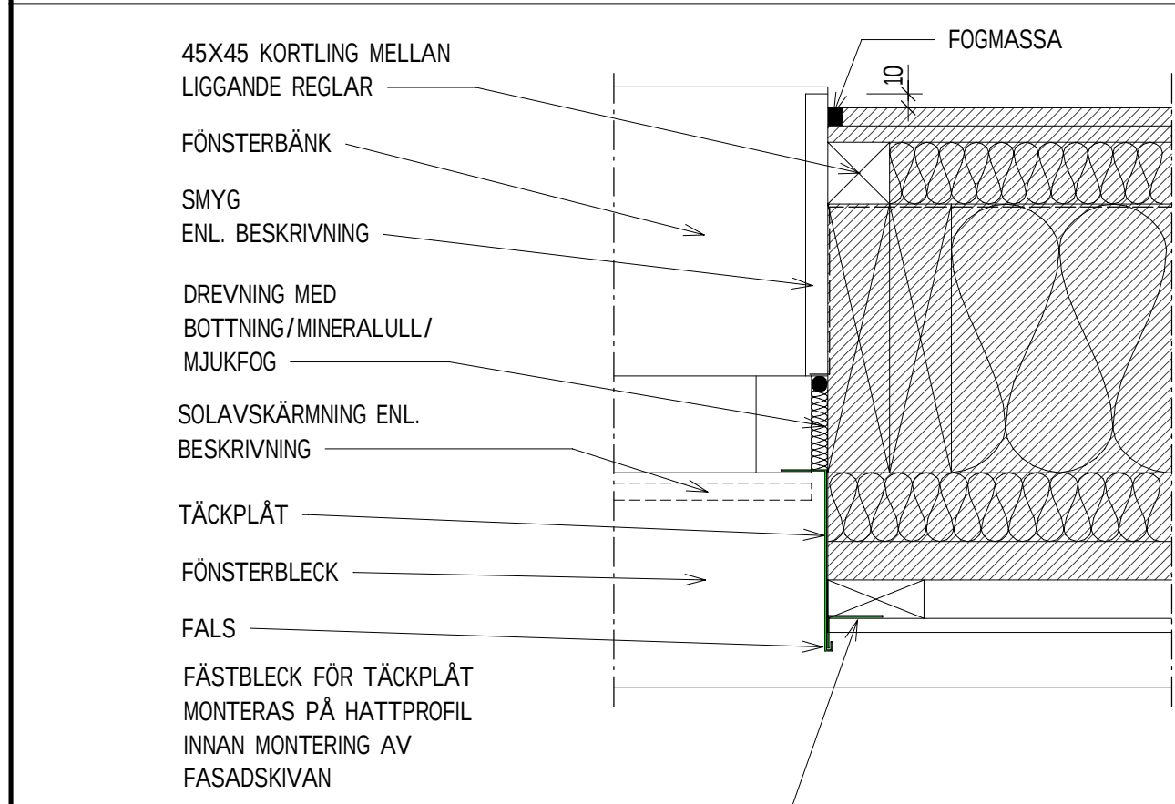
HD2 PRINCIPDETALJ 1:5 FÖNSTER
