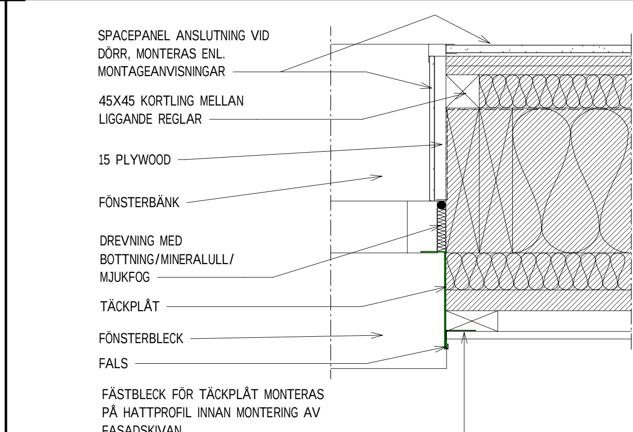
HD3 PRINCIPDETALJ 1:5 FÖNSTER
