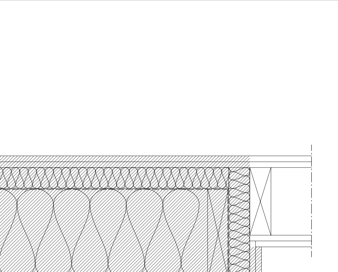
HD13 PRINCIPDETALJ 1:5
