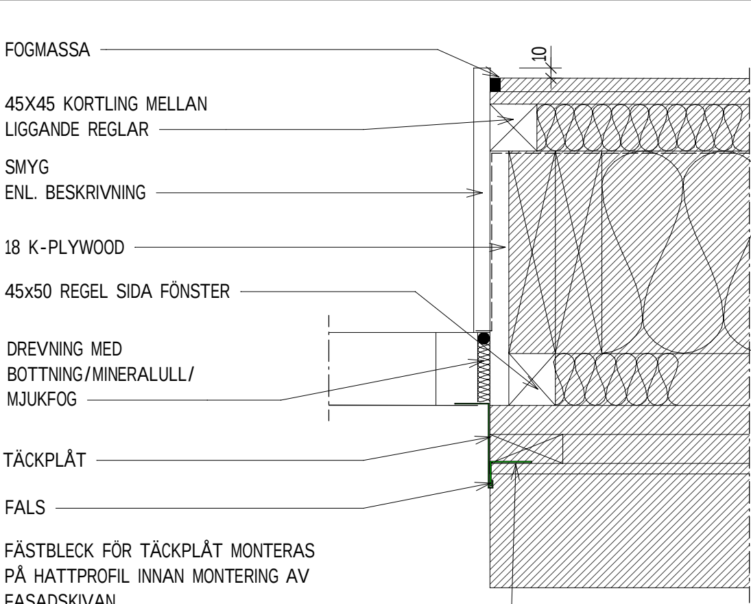
HD7 PRINCIPDETALJ 1:5 METALLPARTI
