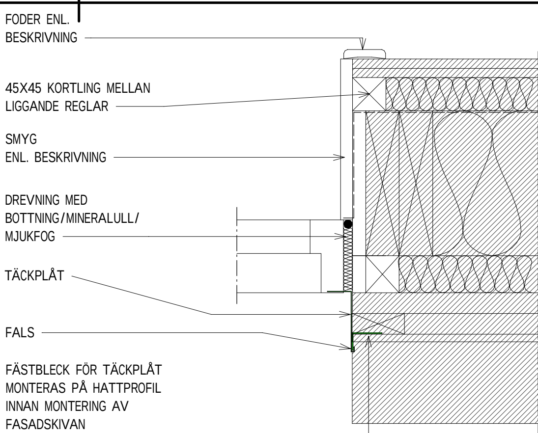
HD9 PRINCIPDETALJ 1:5 STÅLDÖRR
