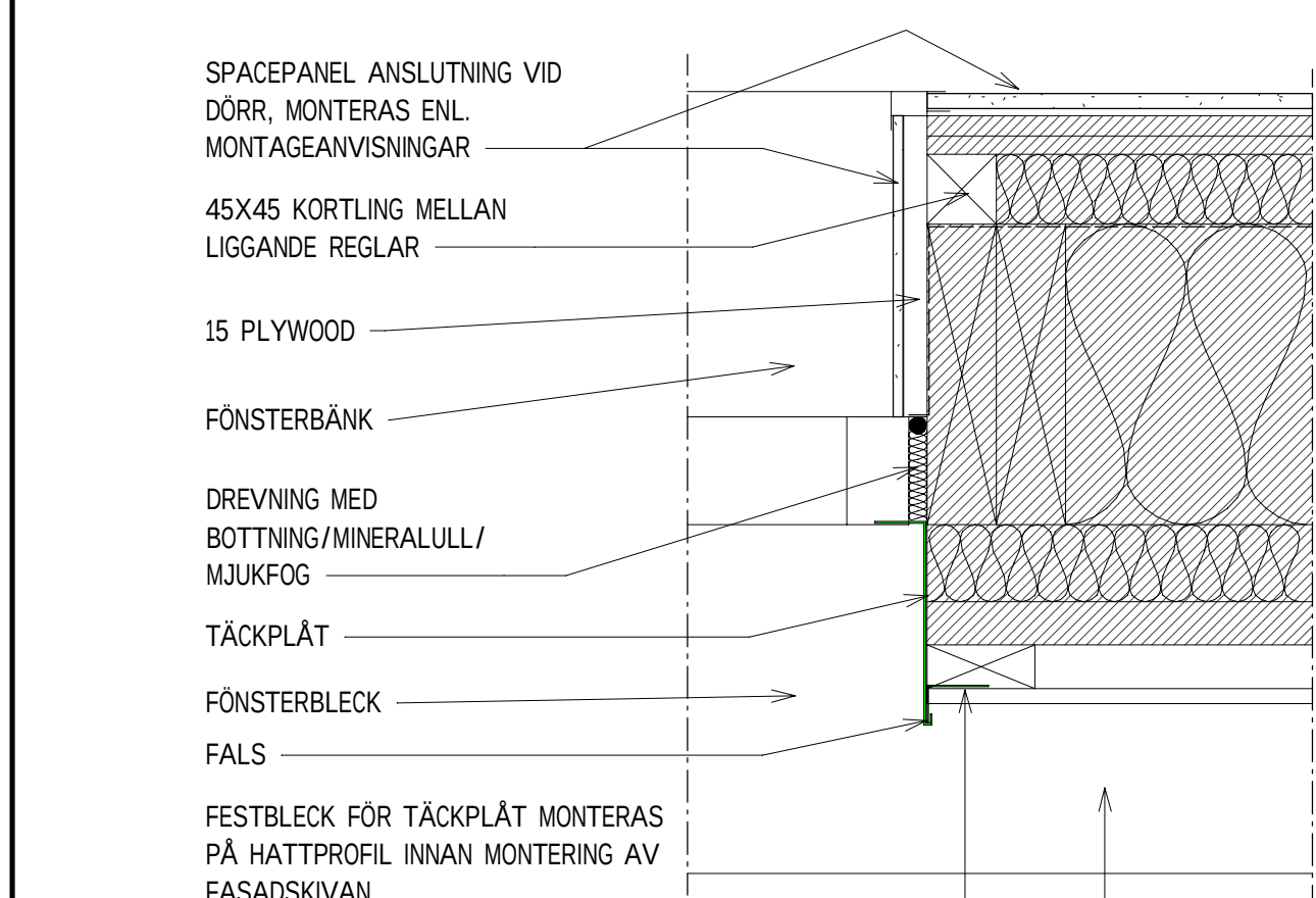
HD4 PRINCIPDETALJ 1:5 FÖNSTER
