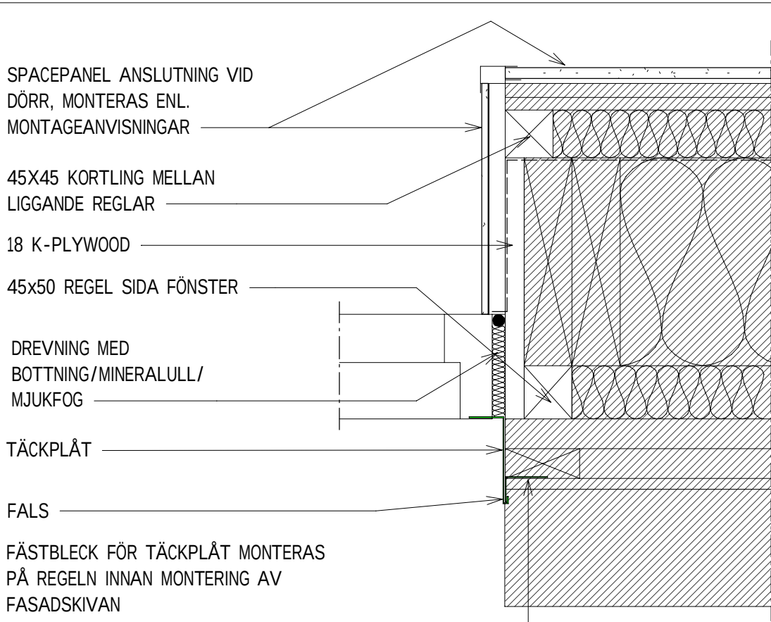
HD10 PRINCIPDETALJ 1:5 STÅLDÖRR
