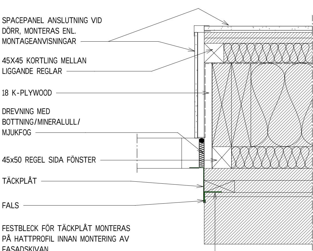
HD8 PRINCIPDETALJ 1:5 METALLPARTI
