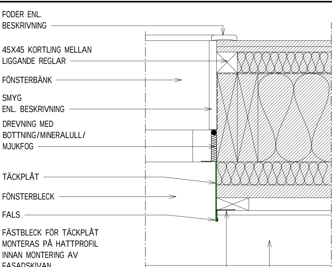
HD5 PRINCIPDETALJ 1:5 FÖNSTER
