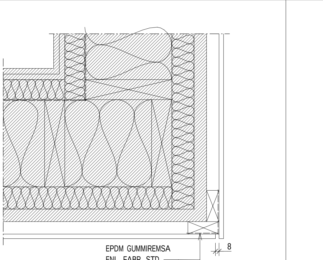
HD14 PRINCIPDETALJ 1:5
