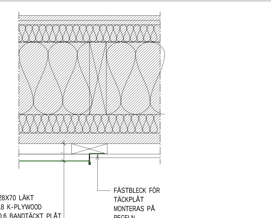
HD13 PRINCIPDETALJ 1:5
