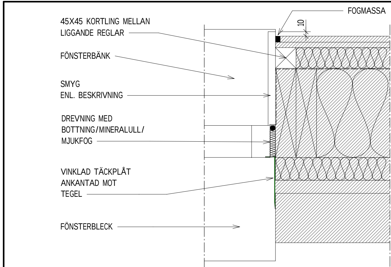
HD1 PRINCIPDETALJ 1:5 FÖNSTER
