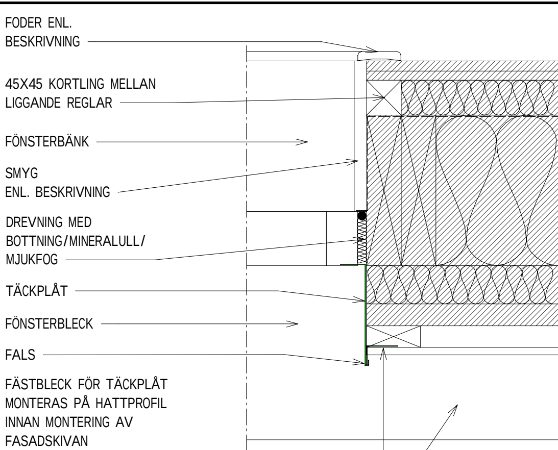
HD16 PRINCIPDETALJ 1:5 FÖNSTER
